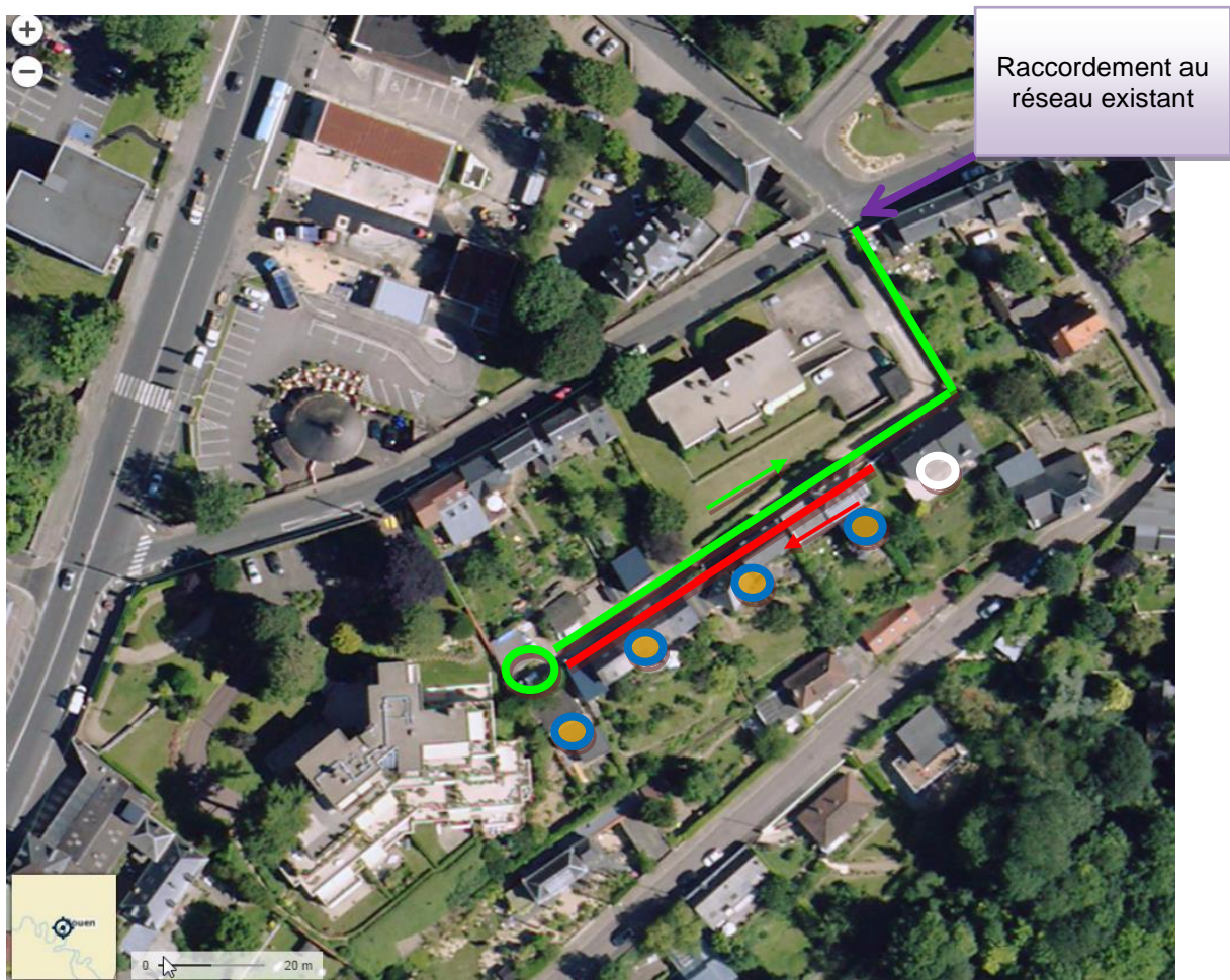
Figure 3 : Représentation graphique de la solution d'assainissement collectif étudiée pour le secteur de l'impasse Herbeuse
